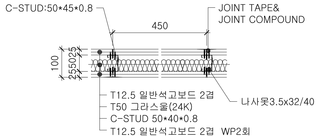
DW2 평면도
