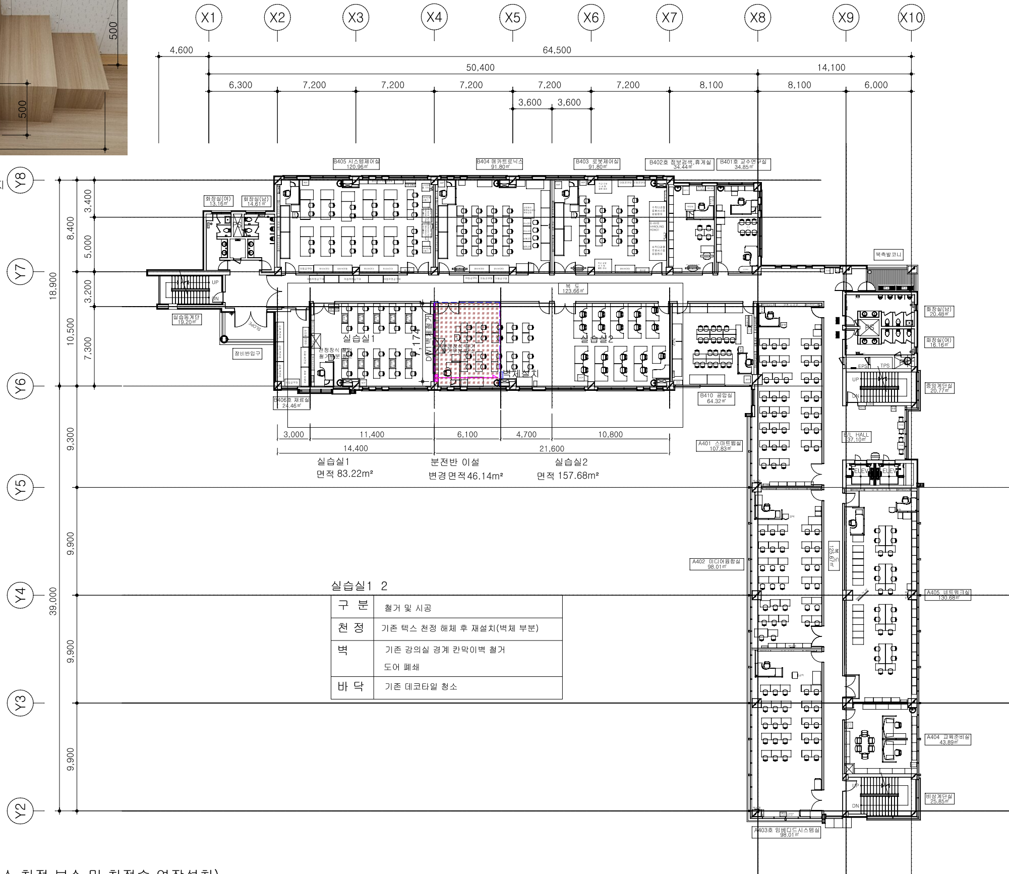
기존 4층평면도
