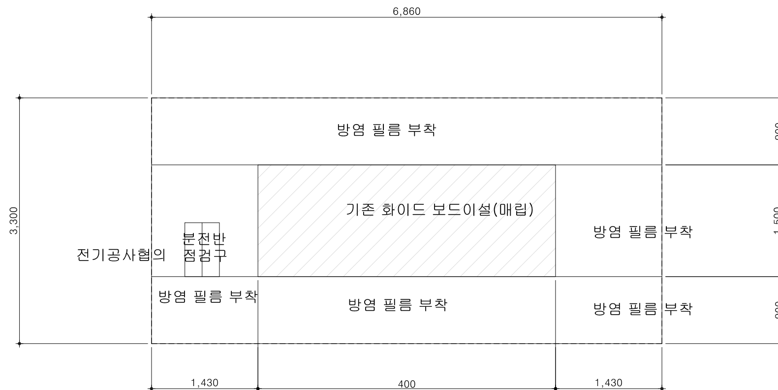
벽체 전개도
